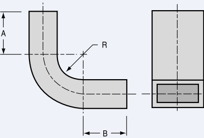
E BEND
